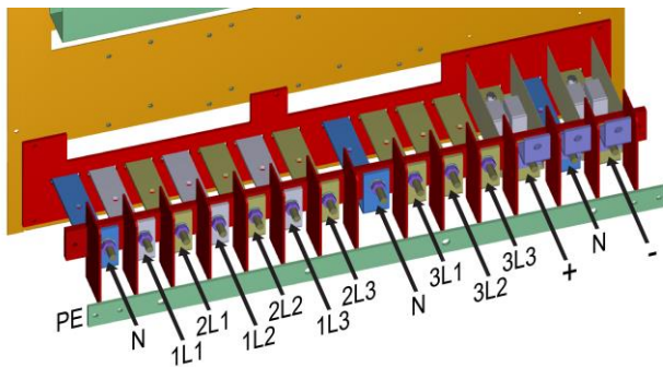
Fig. 2: 120-160-200 kW
