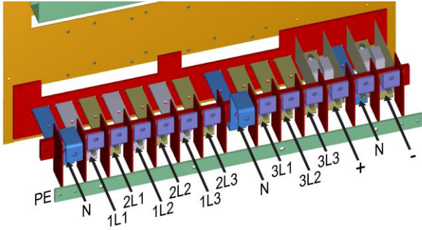
Fig. 3: 250-300 kW
